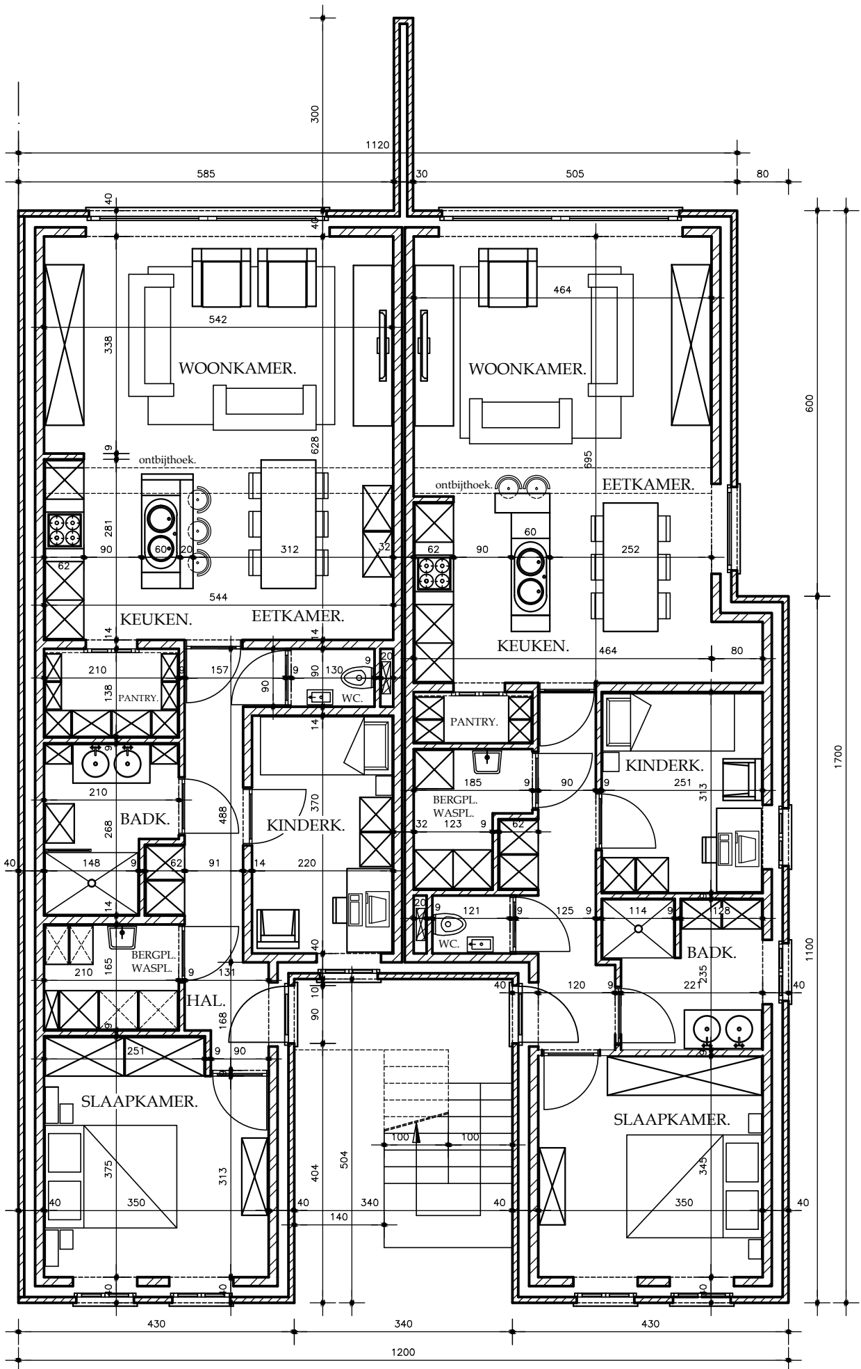
GRONDPLAN.
