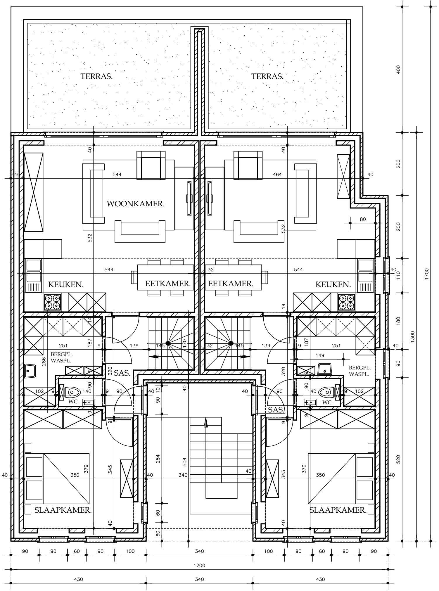
VERDIEPINGSPLAN.
