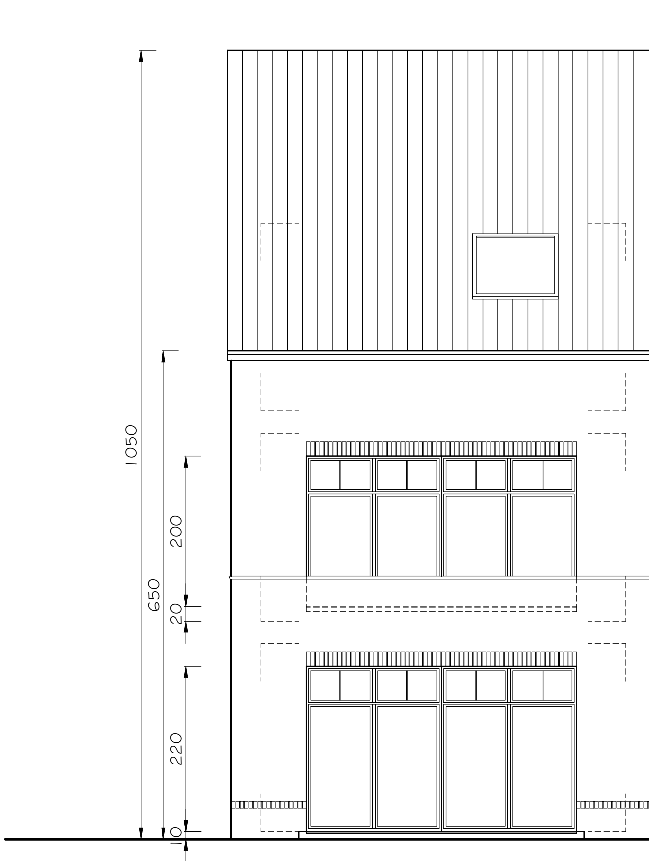
ACHTERGEVEL 1/50
