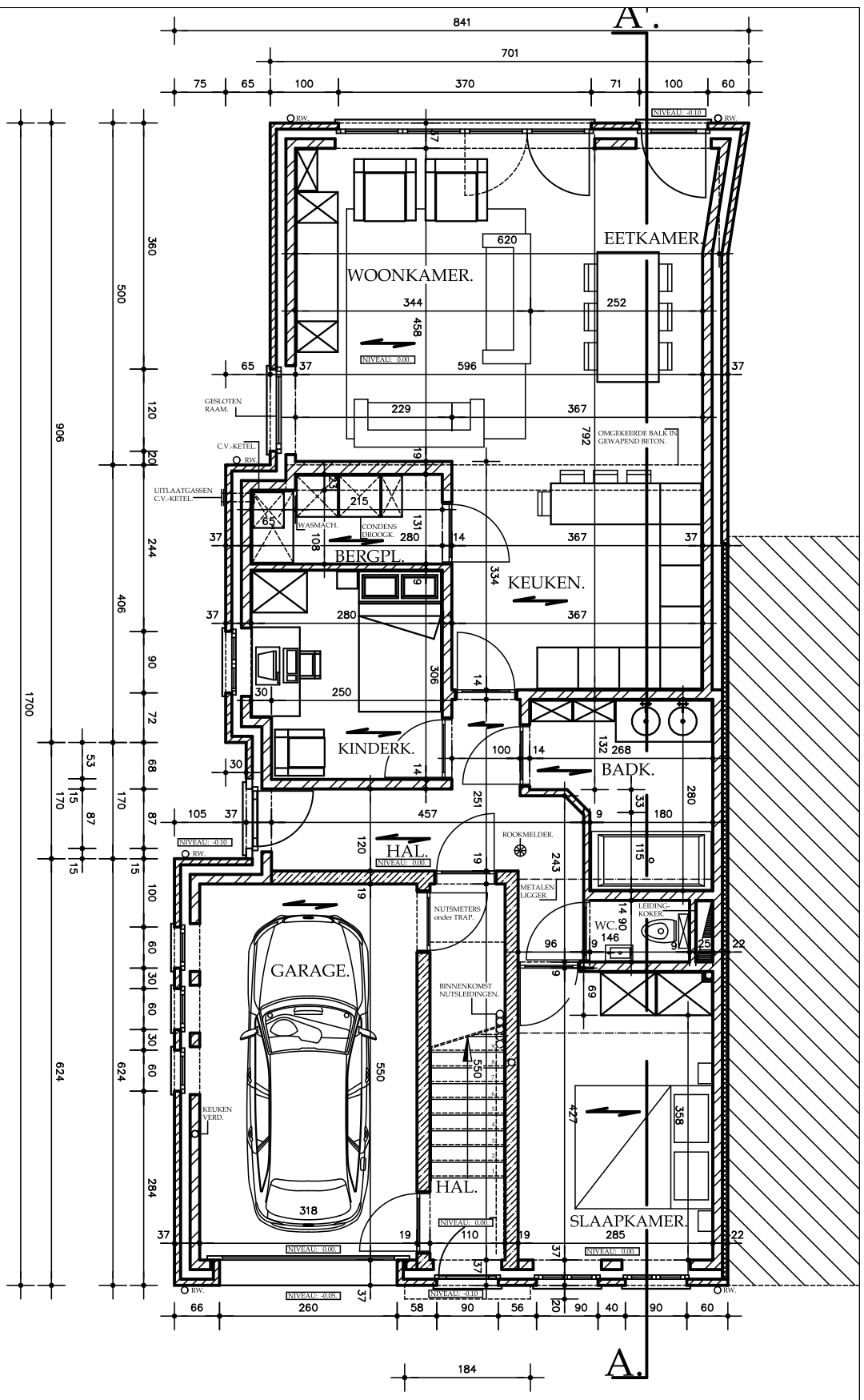
GRONDPLAN.
