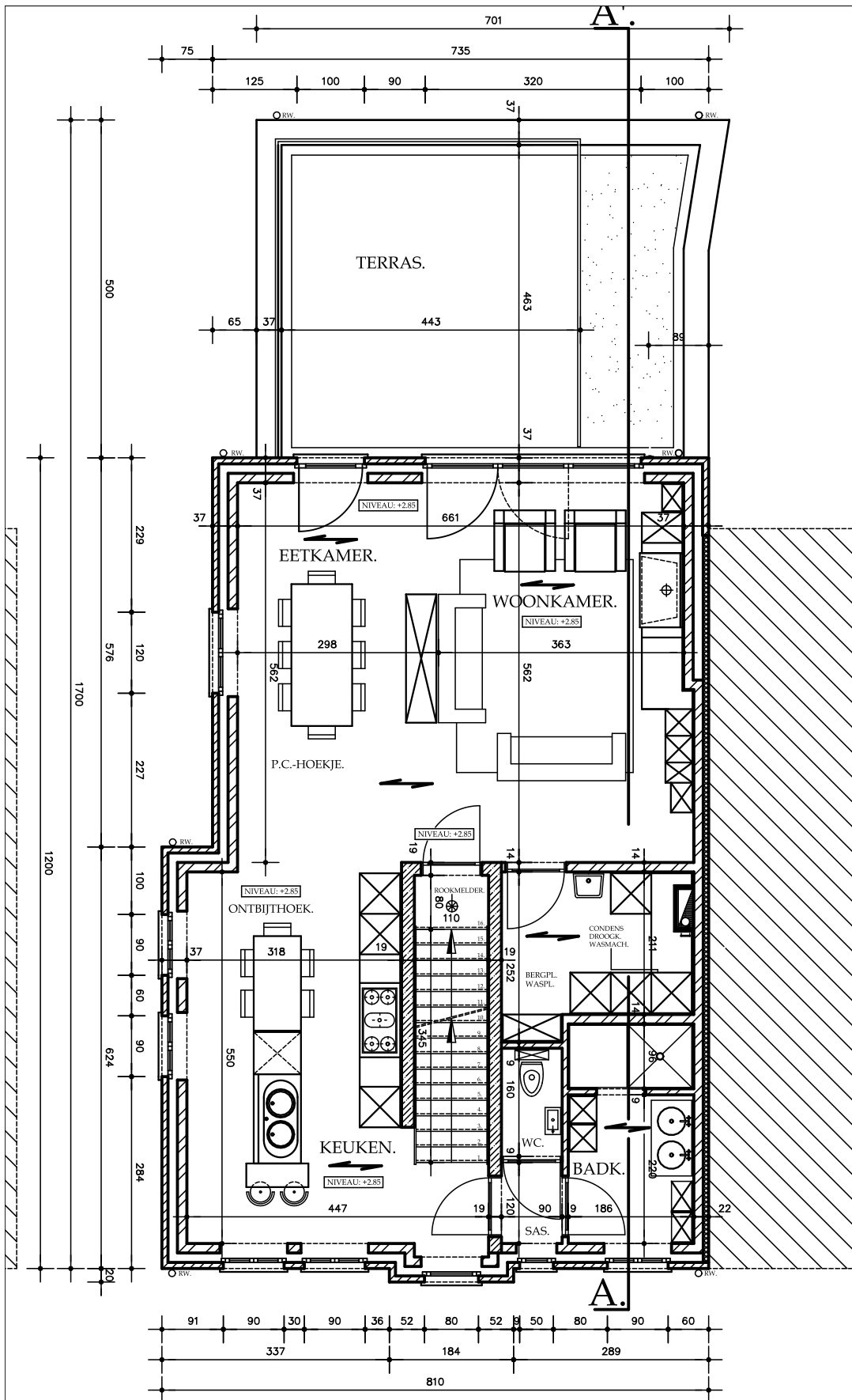
VERDIEPINGSPLAN.
